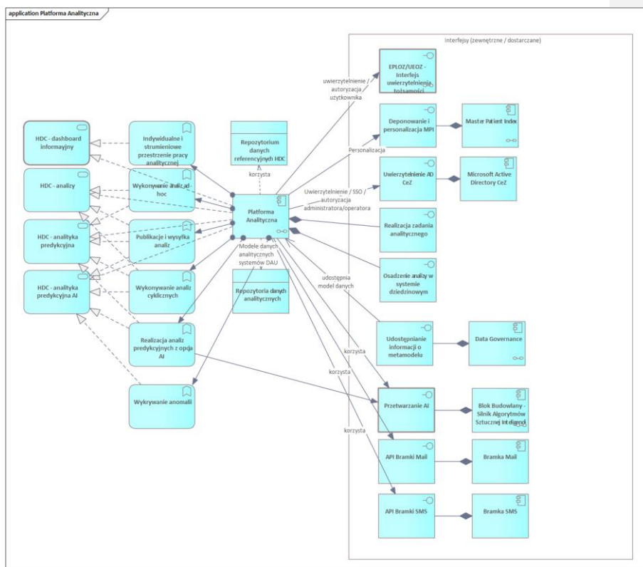
Diagram 6. Struktura komponentu Platforma Analityczna
