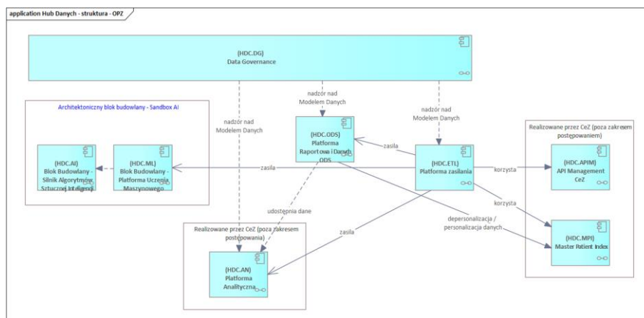
Diagram 2. Struktura Huba Danych CeZ
