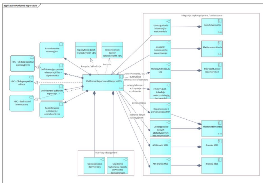
Diagram 5 Struktura komponentu Platforma Danych i Raportowanie ODS
