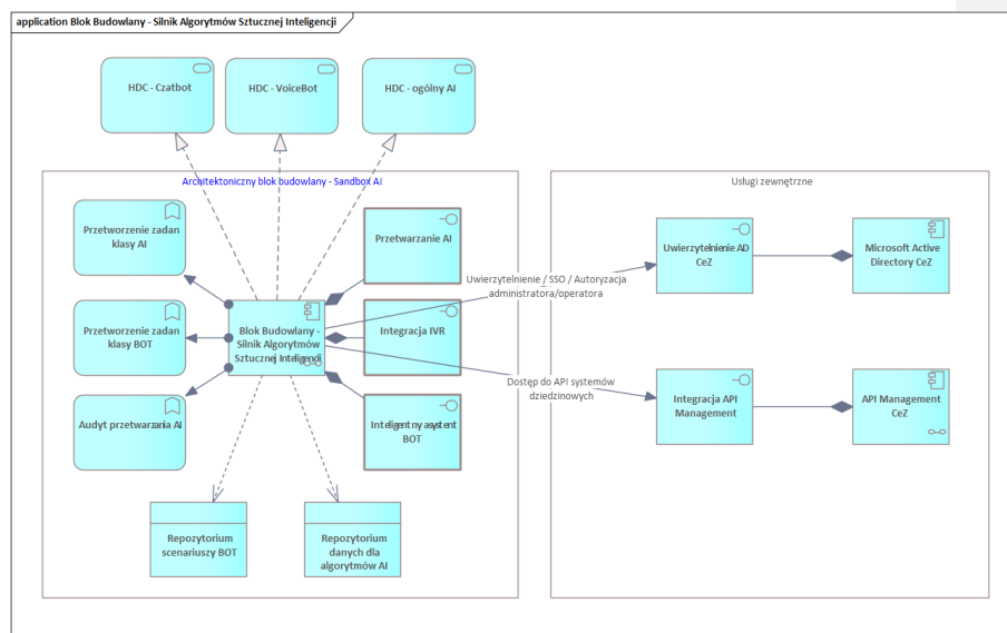
Diagram 8 Struktura komponentu Silnik algorytmów AI (SI)
