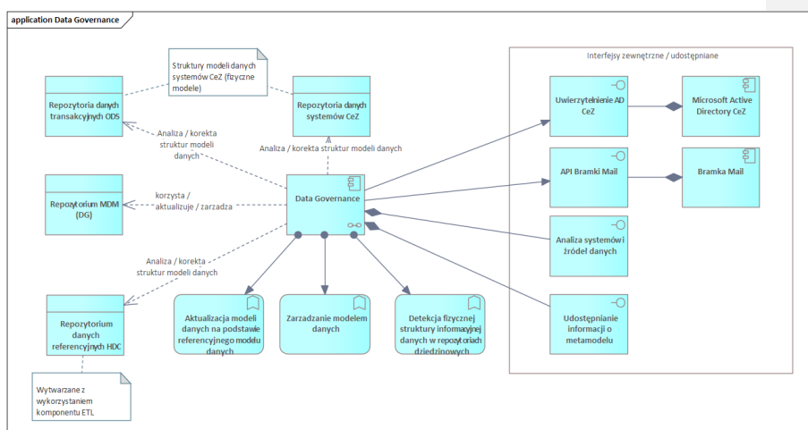
Diagram 3 Struktura komponentu Data Governance
