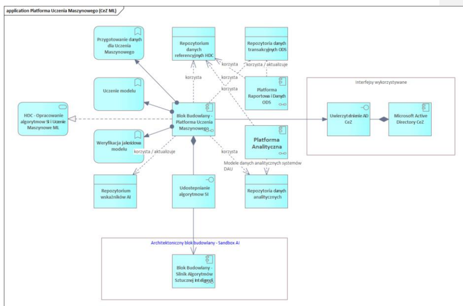
Diagram 7 Struktura komponentów Sandbox AI/ML
